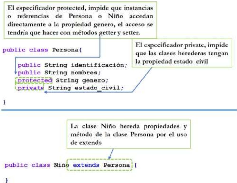
Figura 5 Ejemplo de la Herencia a través de la definición de la clase Persona y Niño.
