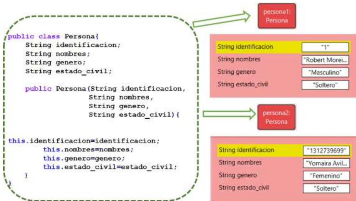
Figura 3 Ejemplo de encapsulamiento a través de la definición de la clase Persona.
