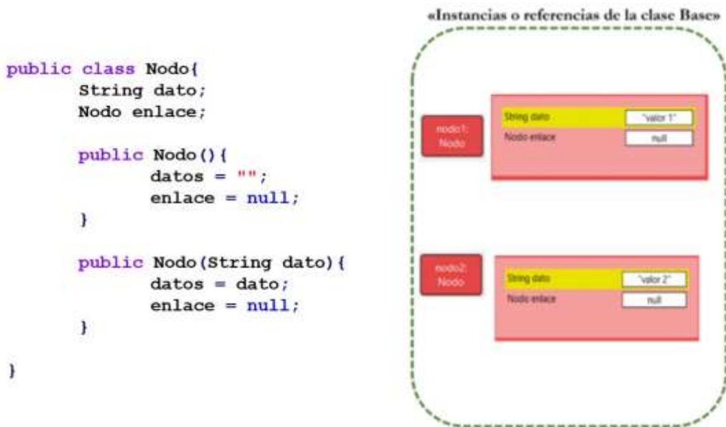
Figura 9 Clases e instancias.
