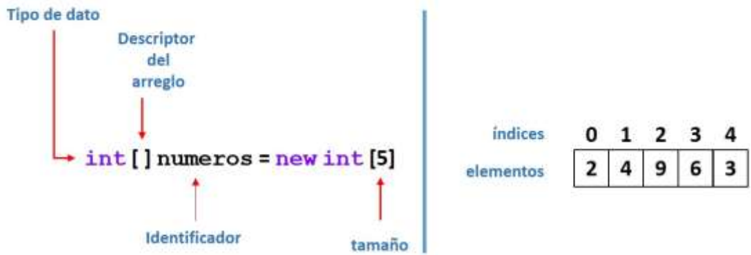
Figura 12 Estructura de un arreglo unidimensional.
