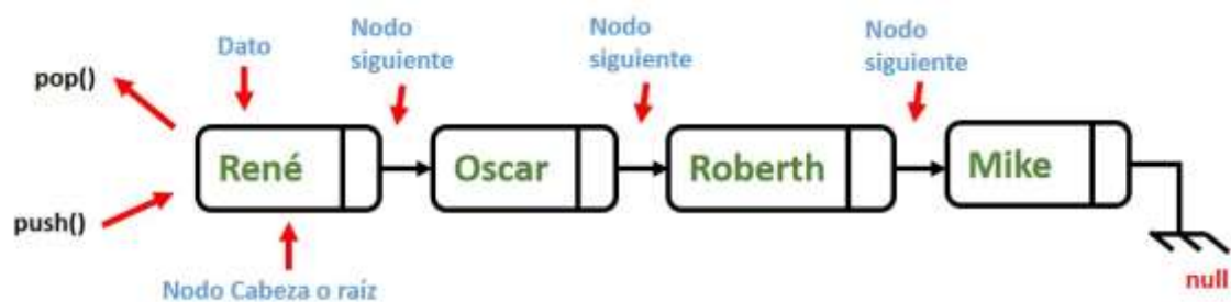
Figura 17 Estructura de una pila
