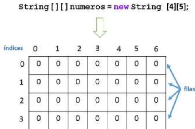
Figura 16 Representación de un arreglo bidimensional.
