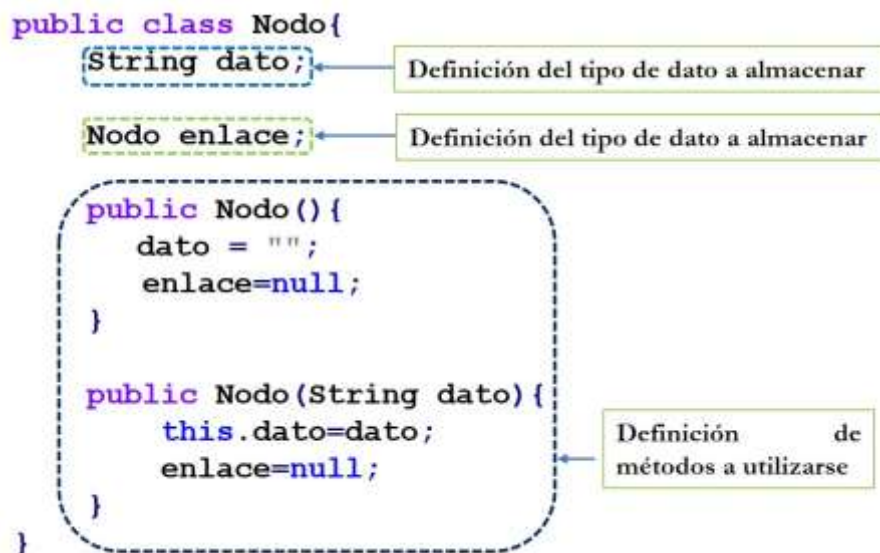
Figura 8 Elementos del tipo de dato abstracto Nodo .
