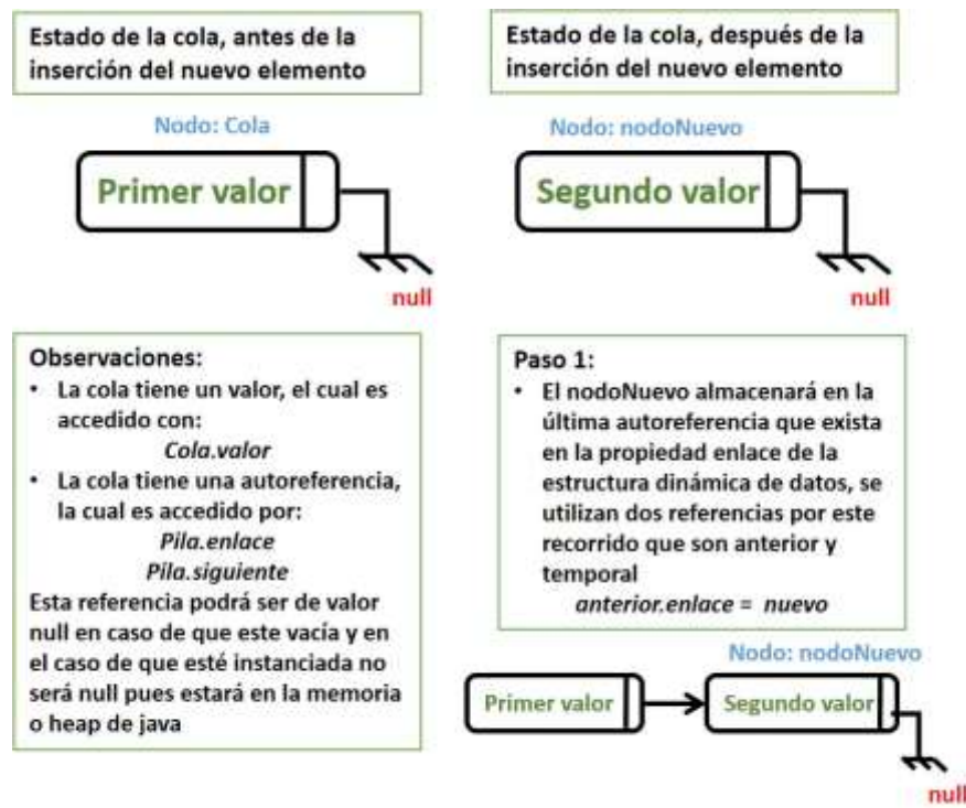
Figura 25 Proceso de inserción en la cola
