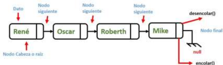
Figura 22 Representación de una cola
