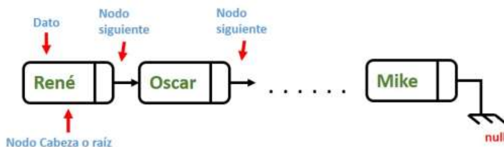
Figura 26 Estructura de una lista simplemente enlazada.
